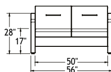
Vue de face
