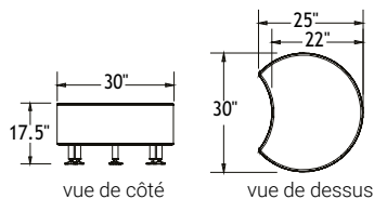
vue de côté
